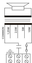
Schaltplan
