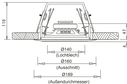
Seitenansicht (Masseinheit: mm)
