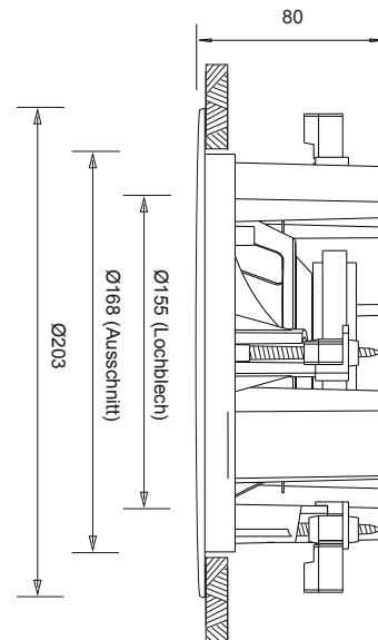
Seitenansicht (Masseinheit: mm)
