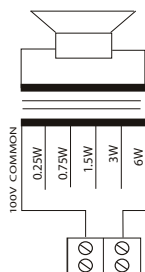
Schaltplan
