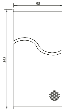
Vue de face (unité de mesure : mm)
