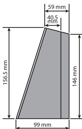
SEITENANSICHT
