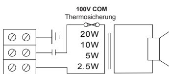
Schaltplan
