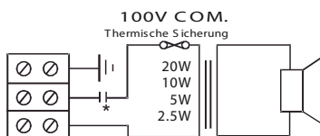
Schaltplan
