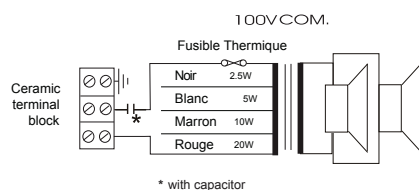
Schéma de branchement
