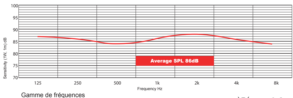
Sensibilité de la bande d'Octave
