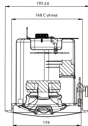
Vue de côté (unité de mesure: mm)
