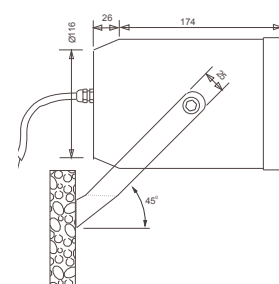
Vue de côté (unité de mesure : mm)
