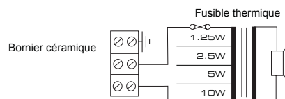
CAD10/TC Schéma de branchement du commun 100 V
