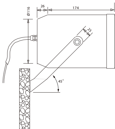
Vue de côté (unité de mesure : mm)
