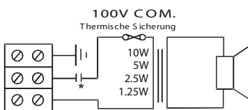
Schaltplan
