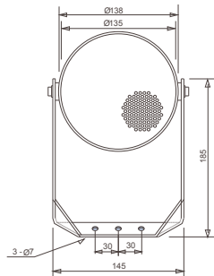
Vue de face (unité de mesure : mm)
